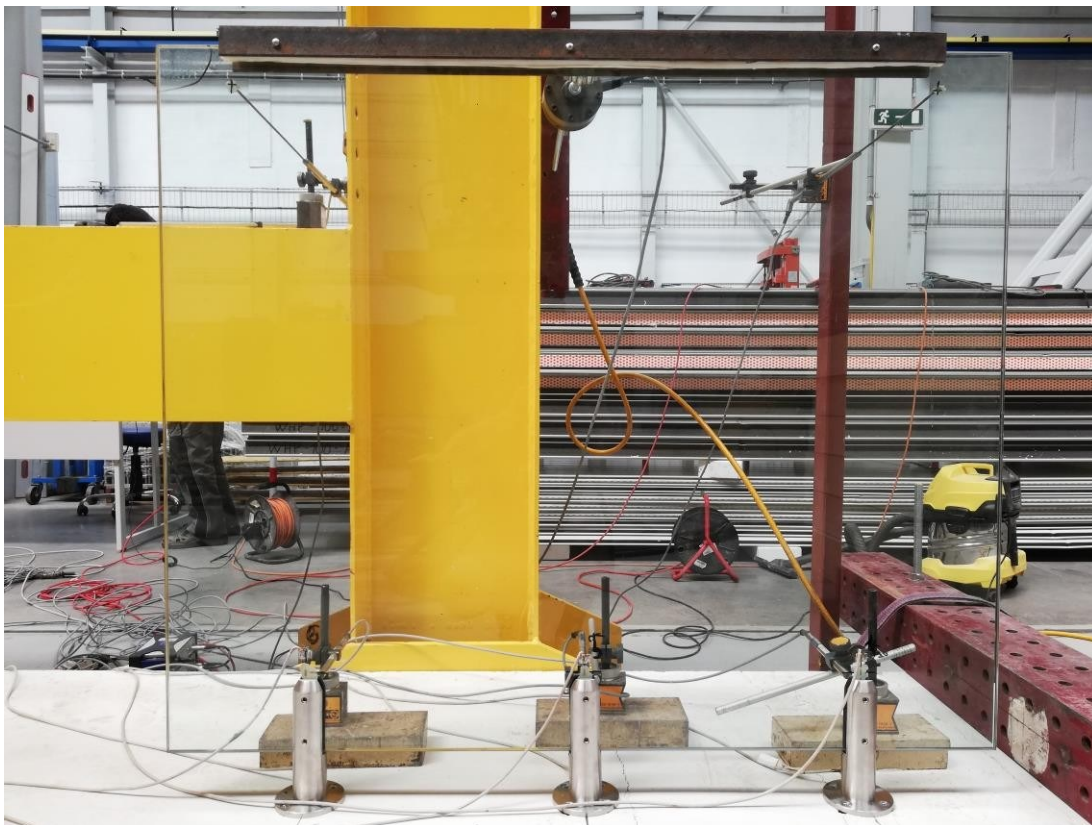
Baugruppe 3x SPIGOT
