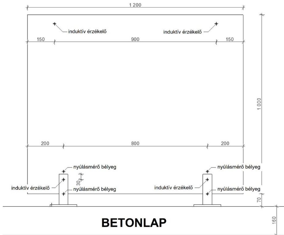
2x SPIGOT SZETT ÁBRÁJA
